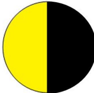
Dernier quartier
