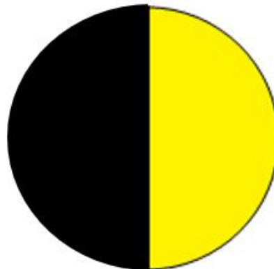
Premier quartier
