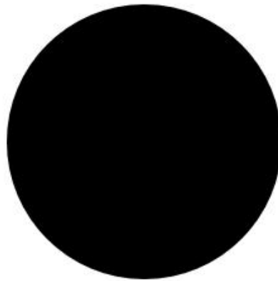
Nouvelle lune
