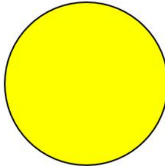
Pleine lune
