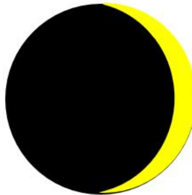
Premier croissant
