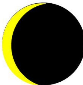
Premier croissant
